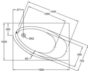
RENOVA NR. 1 Asymmetrische Eckwanne links Mod.- Nr. 65 73 40 03.03.2008/Re-Th
